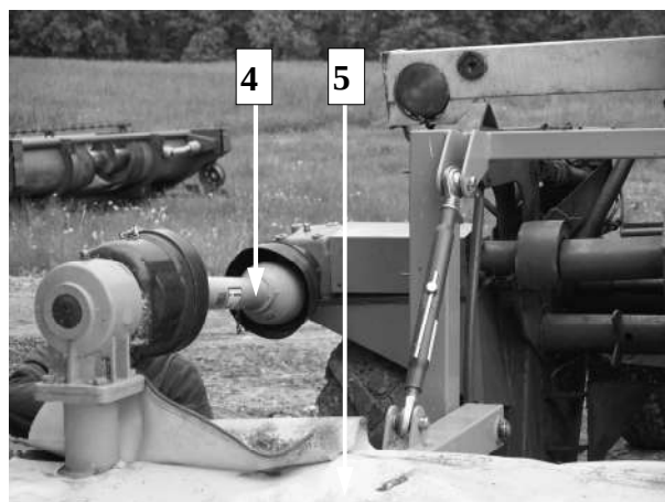
Рис. 7. Навешивание косилки KDF 390 на машину «Fortschritt»
