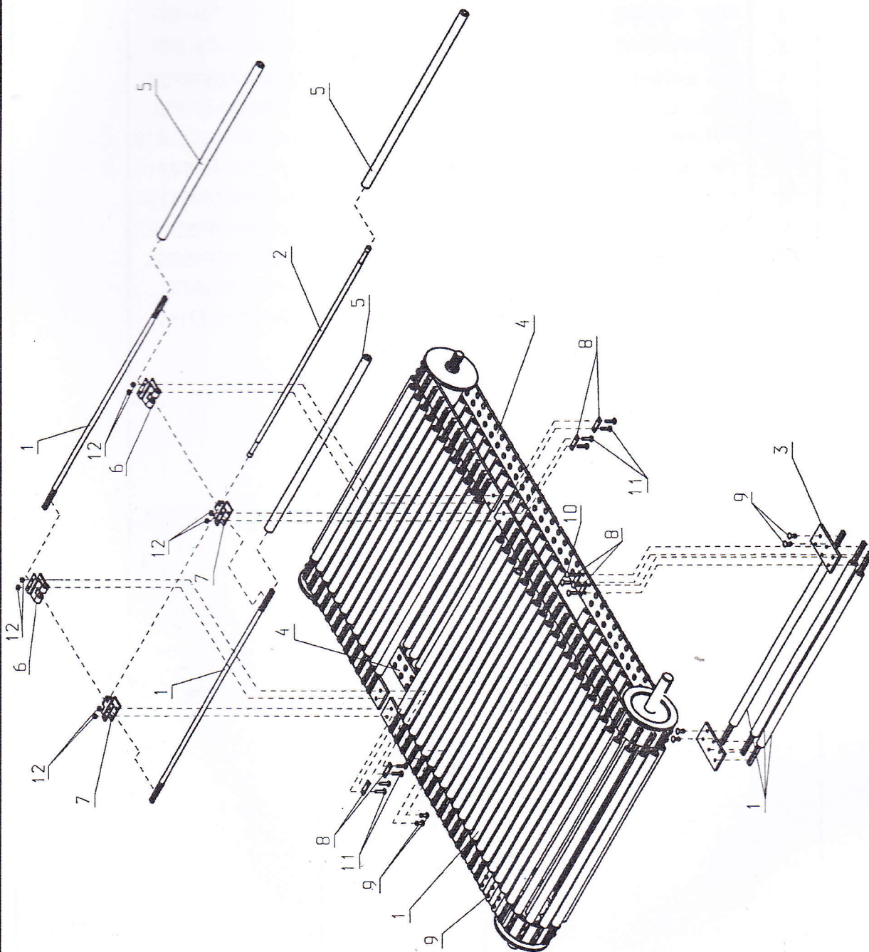
Tablica T-10 Przenośnik stołu przebiecznego
