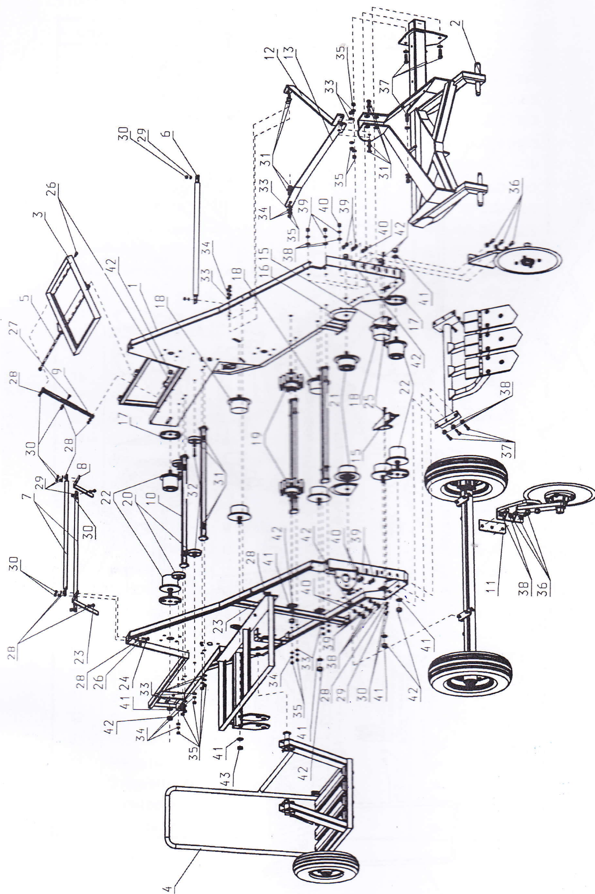
Tablica T-2. Rama kpl.
