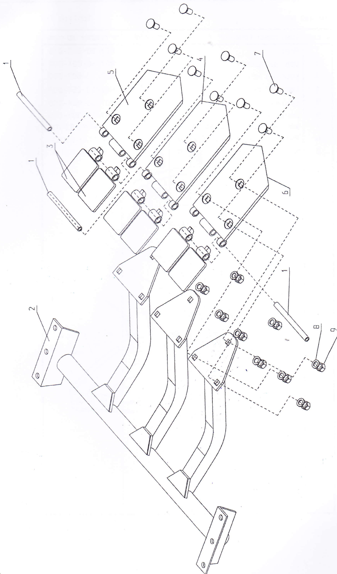
Tablica T-7 Lemiesz kpl.
