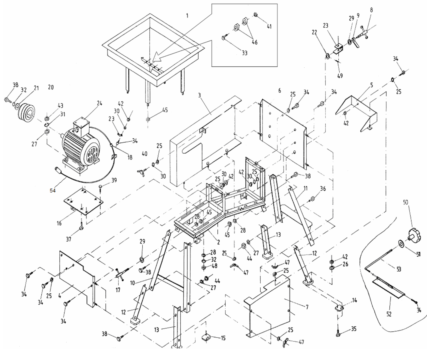
Tablica 1 Zgniatacz ziarna SIPMA ZZ 7510 TYTAN 8752-000-000.00
