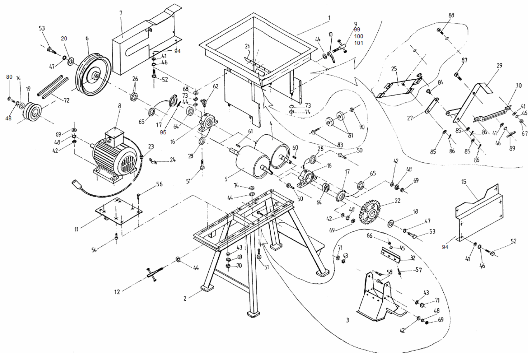
Tablica 1 Zgniatacz ziarna SIPMA ZZ 7500 TYTAN 8733-000-000.00
