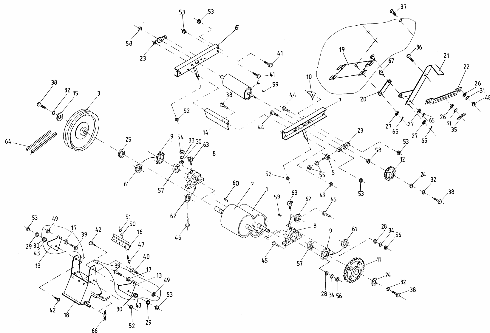
Tablica 2 Zgniatacz ziarna SIPMA ZZ 7510 TYTAN 8752-000-000.00
