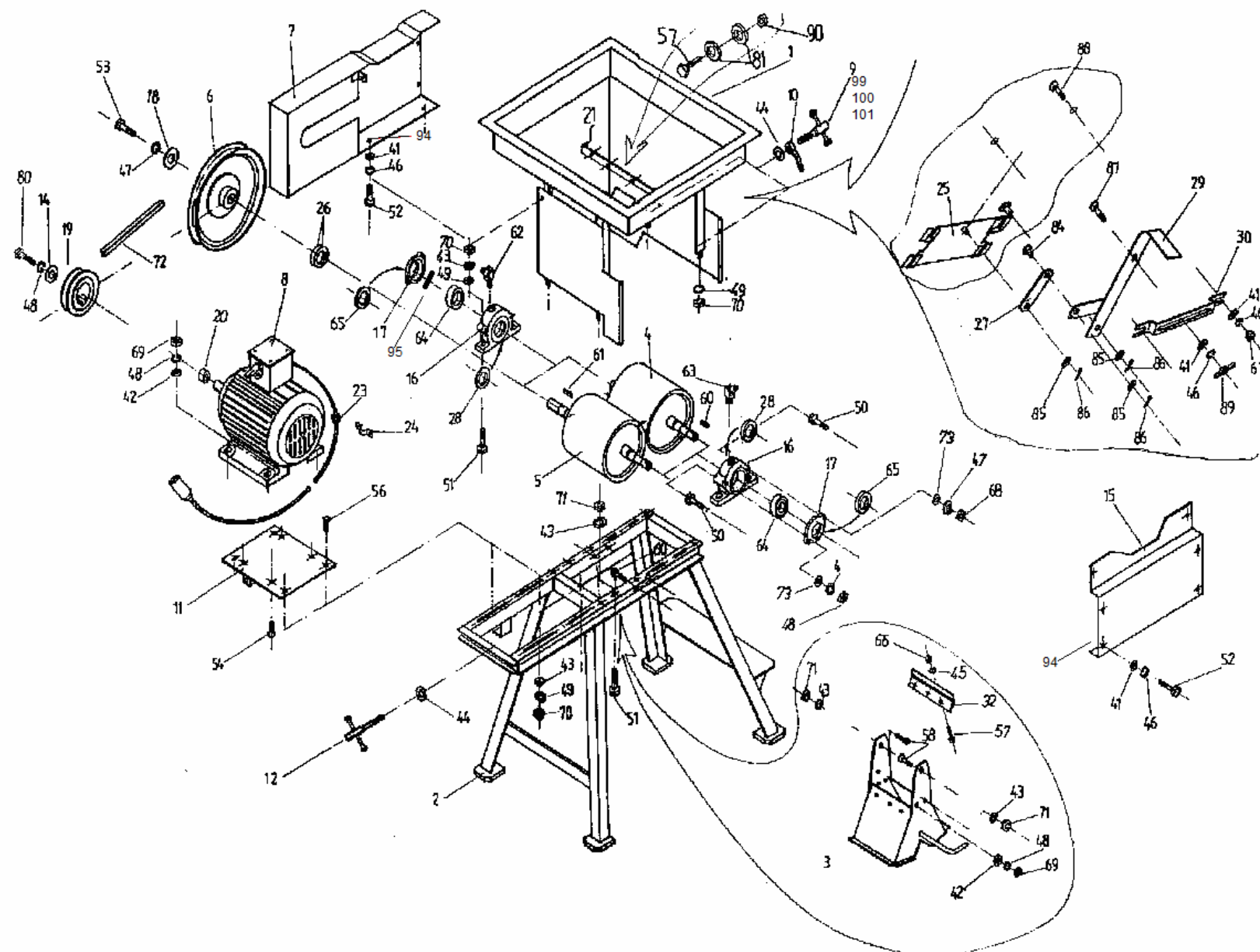
Tablica 1 Zgniatacz ziarna SIPMA ZZ 4000 TYTAN 8730-000-000.00
