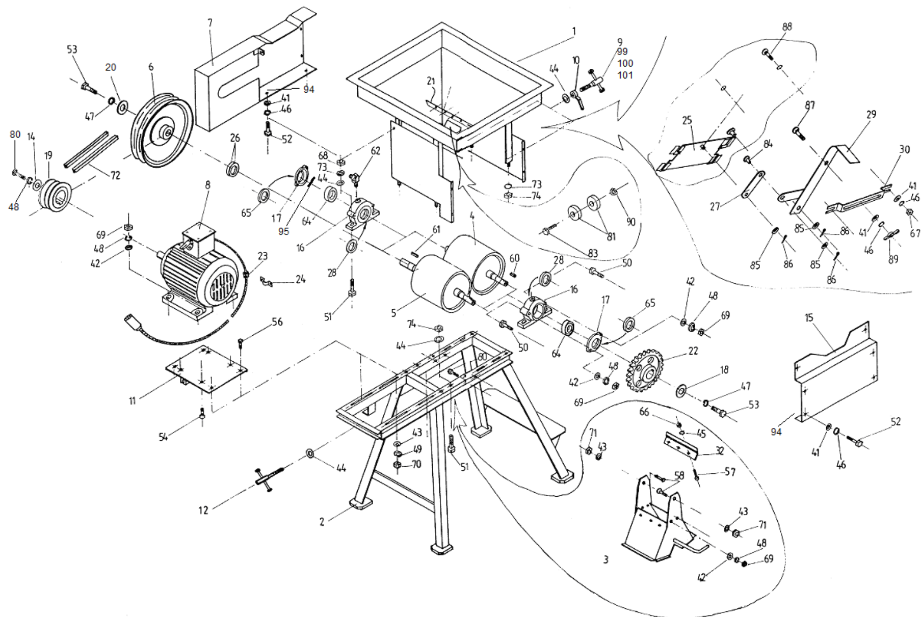
Tablica 1 Zgniatacz ziarna SIPMA ZZ 7520 TYTAN 8733-000-000.00
