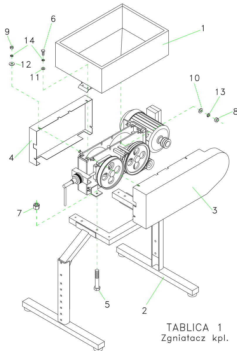
Tablica 1 Zgniatacz ziarna kpl. 8759-000-000.00
