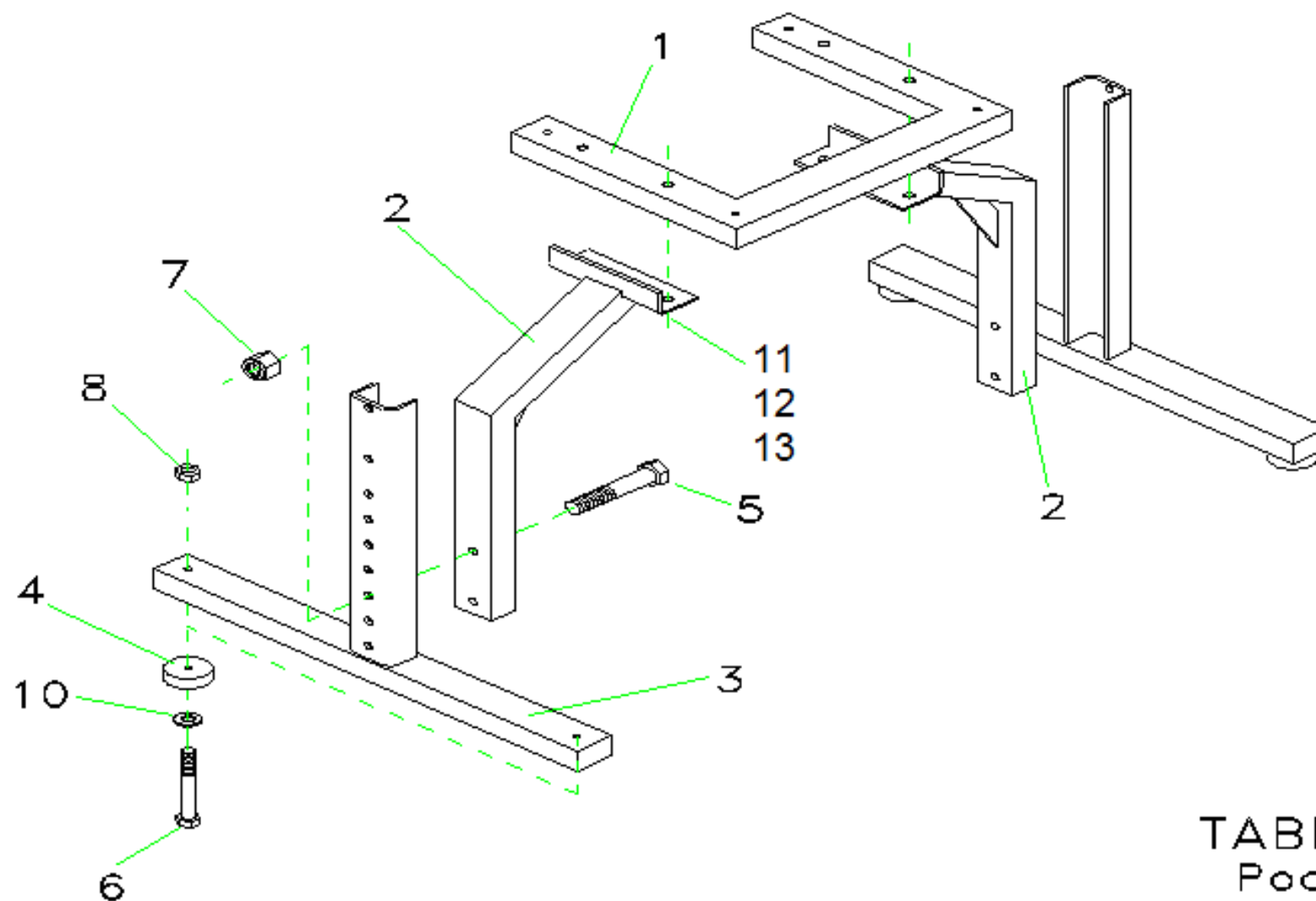
Tablica 3 Podstawa 8759-040-500.00
