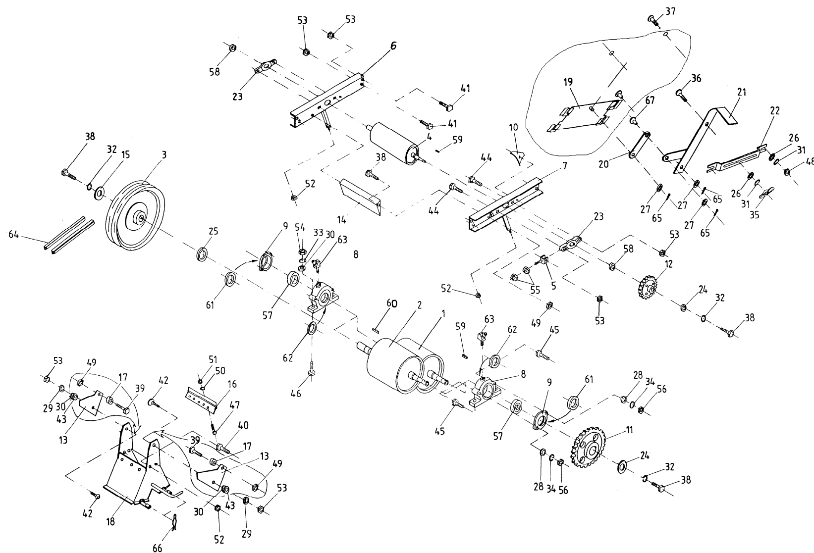
Tablica 2 Zgniatacz ziarna SIPMA ZZ 7530 TYTAN 8752-000-000.00
