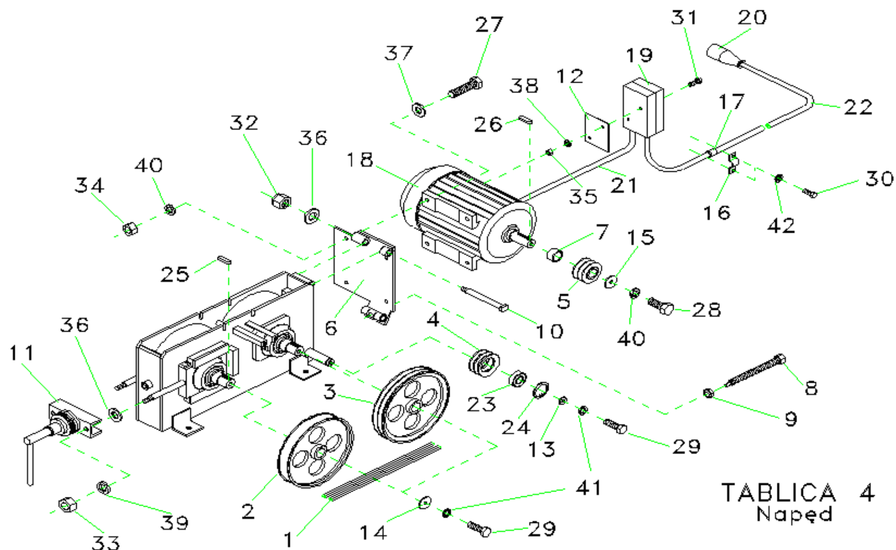
Tablica 4 Napęd
