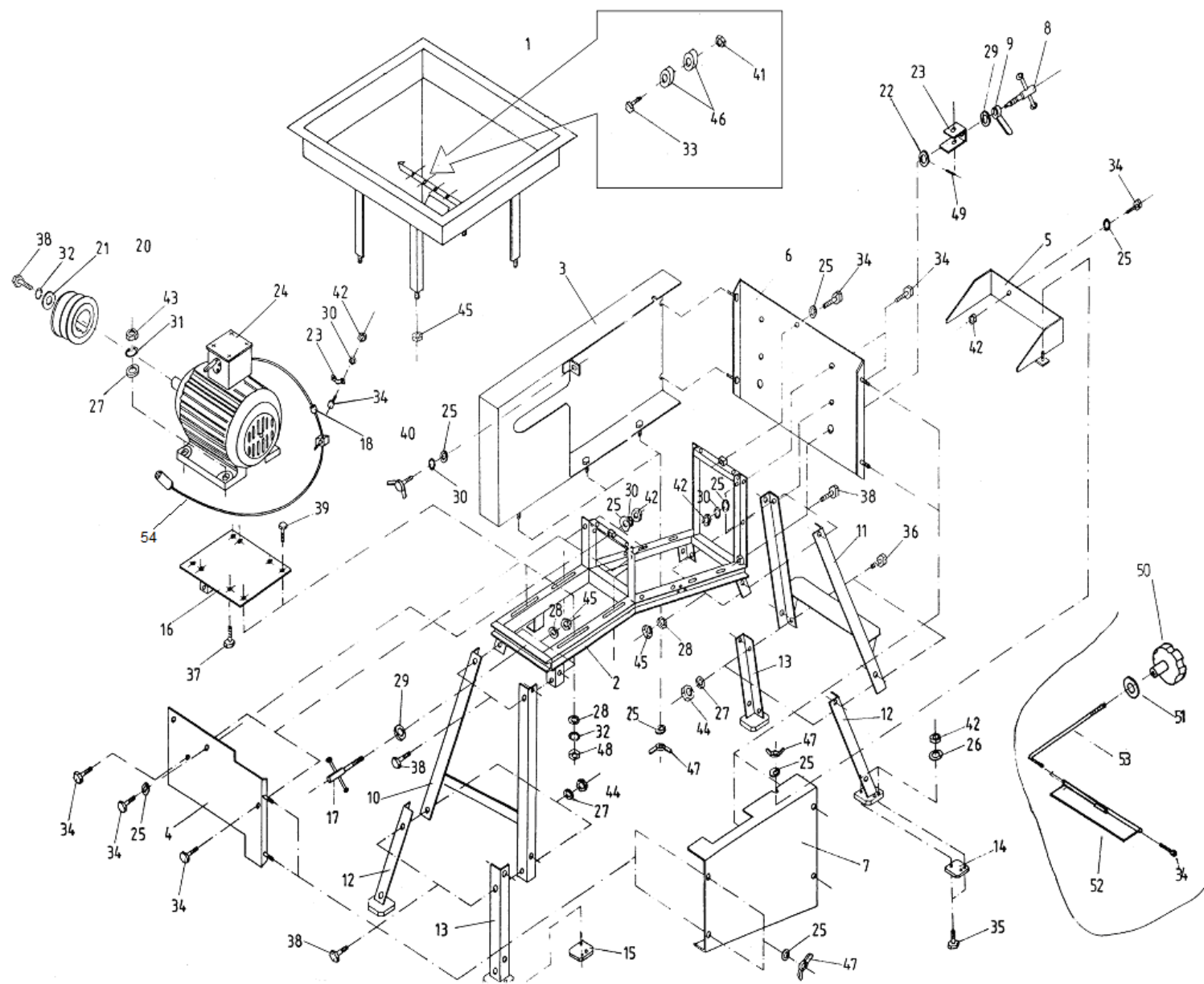
Tablica 1 Zgniatacz ziarna SIPMA ZZ 7530 TYTAN 8752-000-000.00
