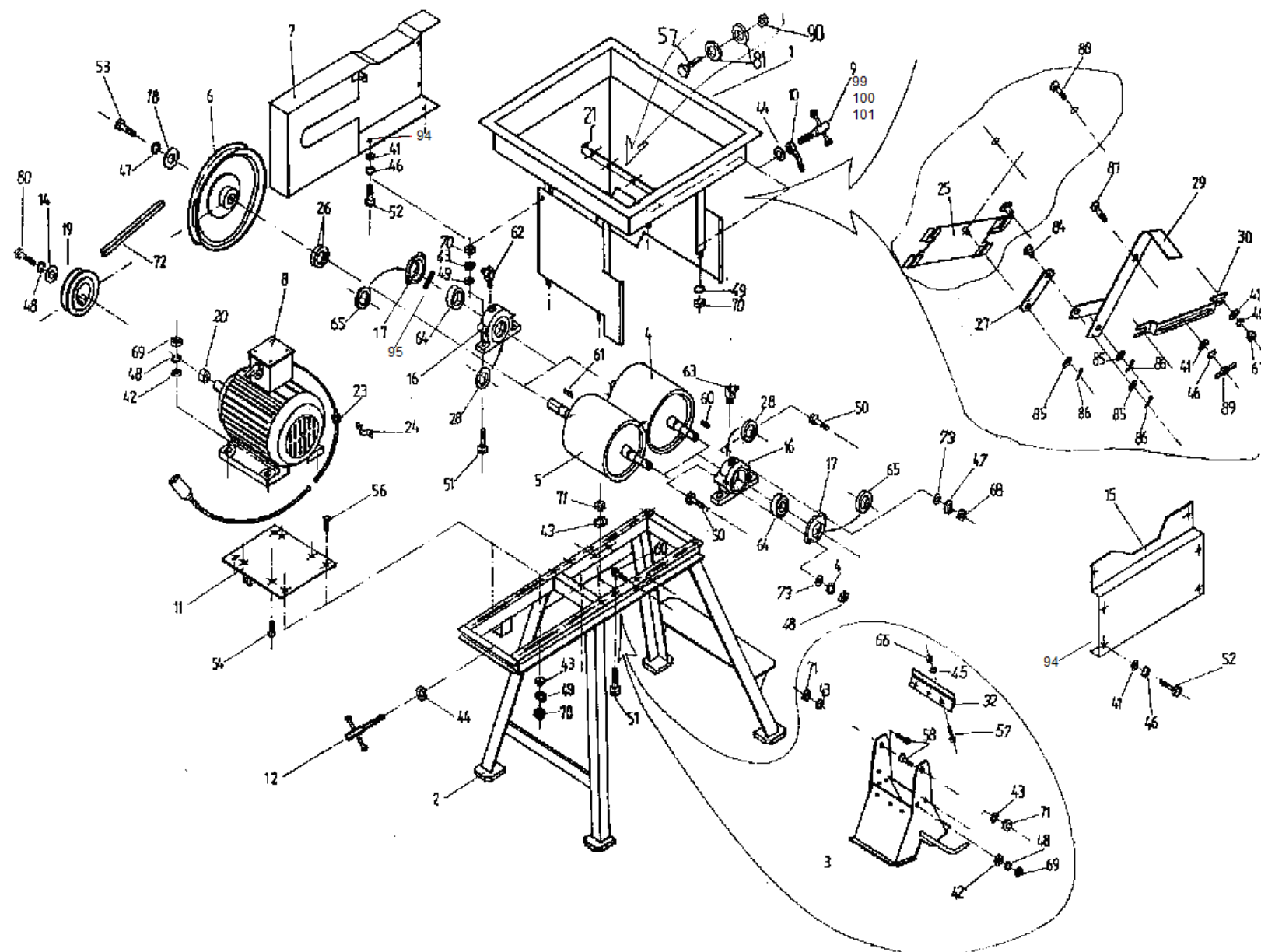
Tablica 1 Zgniatacz ziarna SIPMA ZZ 4020 TYTAN 8730-000-000.00
