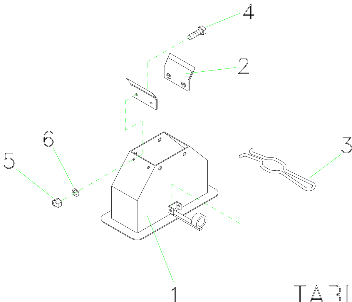
Tablica 7 Zbierak kpl. 8759-030-500.00
